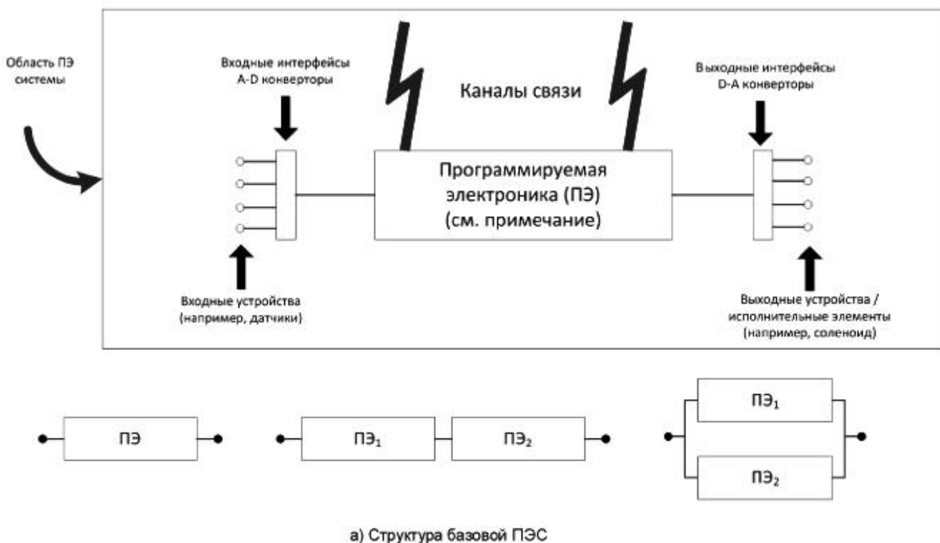
Рисунок 2 - Структура программируемой электронной системы
