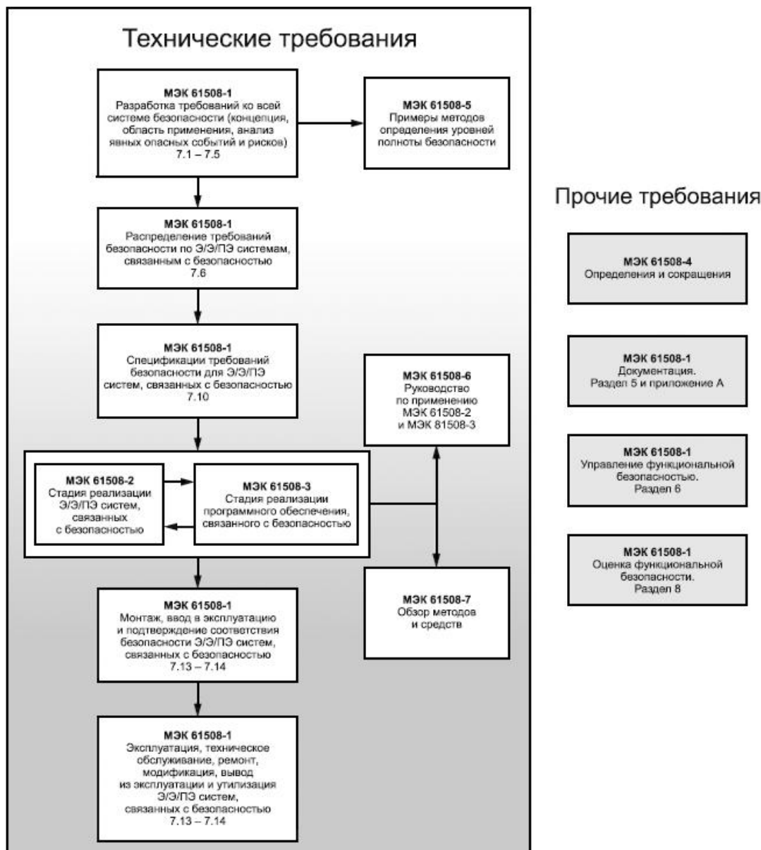
Рисунок 1 - Общая структура серии МЭК 61508
