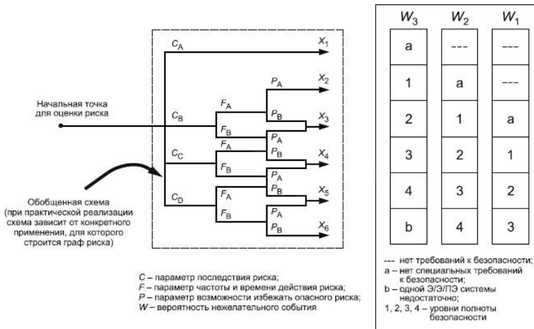
Рисунок Е.1 - Граф риска: общая схема
