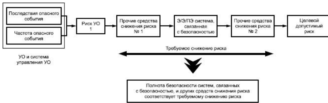
Рисунок А.2 - Понятия риска и полноты безопасности
