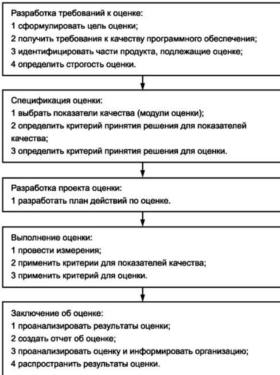
Рисунок 3 - Процесс оценки качества программного продукта
